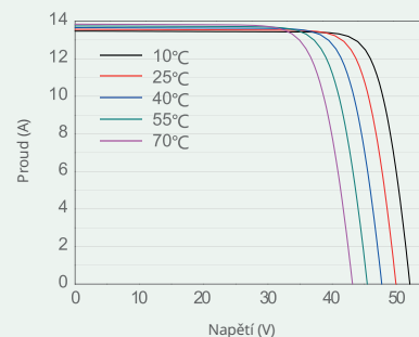
Křivka proudu a napětí (SP540M-72HB)
