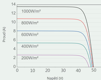
Křivka proudu a napětí (SP540M-72HB)
